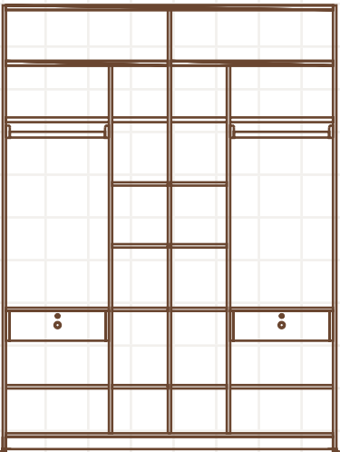
SA W : 1800,2000,2200 D : 600 H : 1950 - 2100 - 2400
