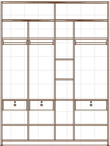
SB W : 1800,2000,2200 D : 600 H : 1950 - 2100 - 2400
