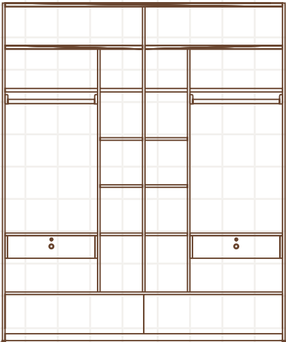
SE W : 1800,2000,2200 D : 600 H : 1950 - 2100 - 2400
