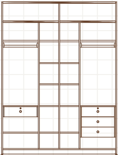
SC W : 1800,2000,2200 D : 600 H : 1950 - 2100 - 2400
